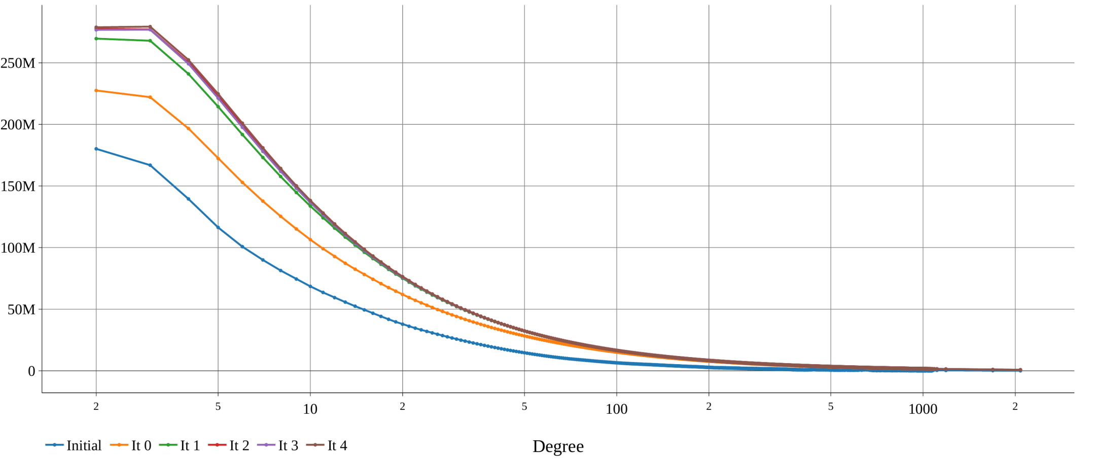
N2N AID, clueweb09
