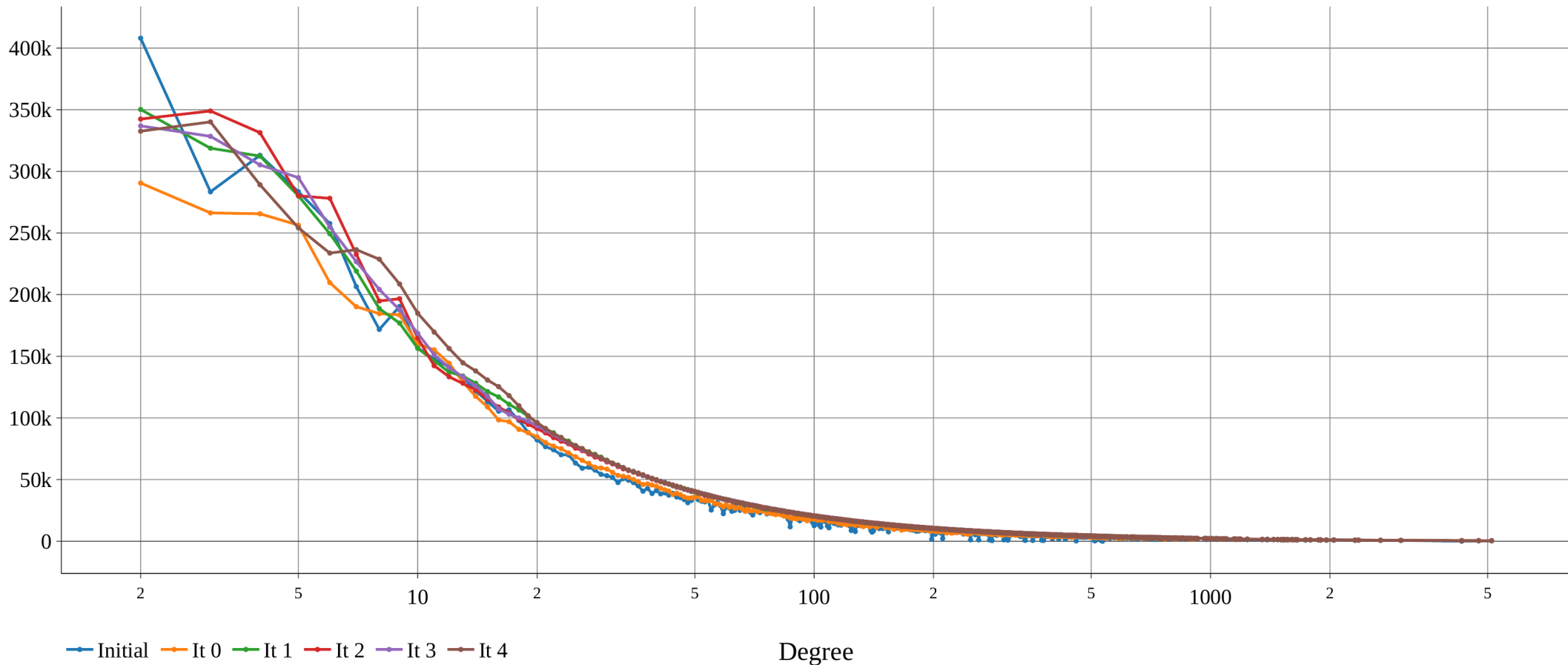
N2N AID, warwiki_csr
