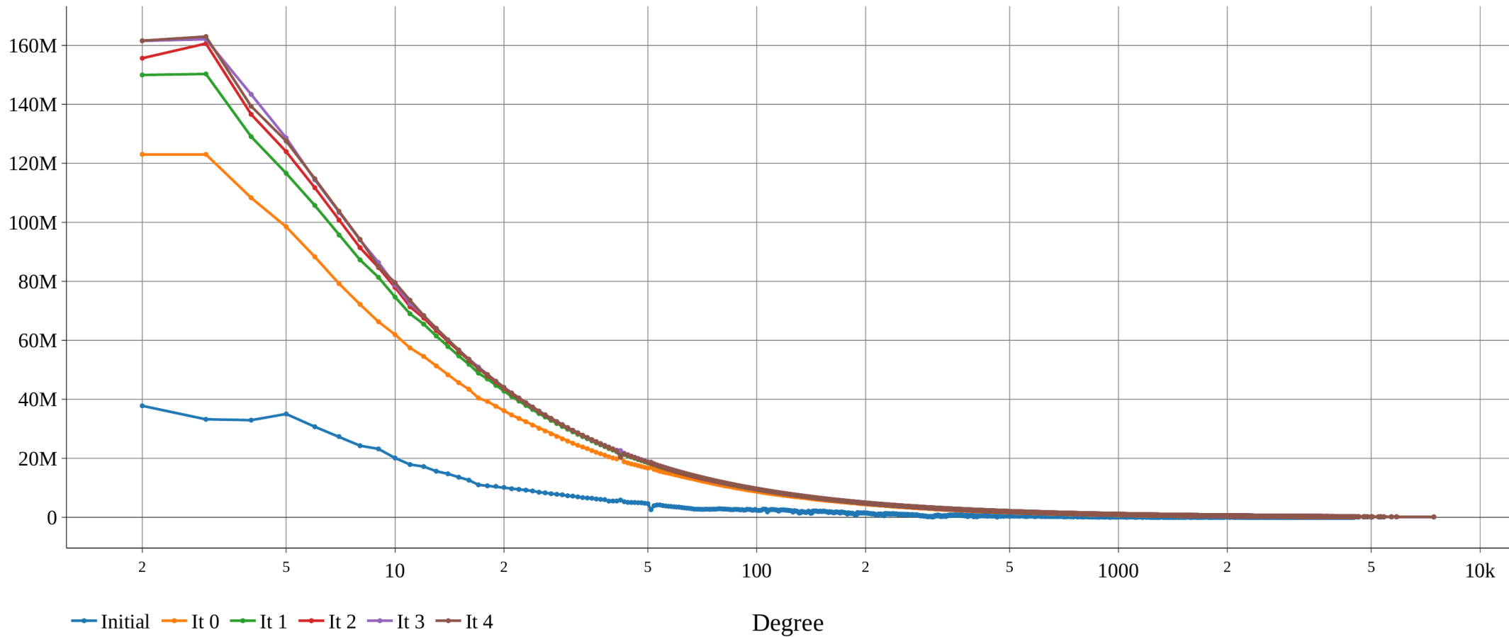
N2N AID, clueweb12
